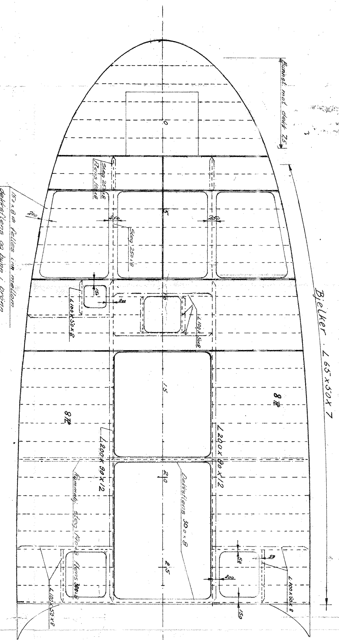
Hoveddekk (Akkorddekk)
