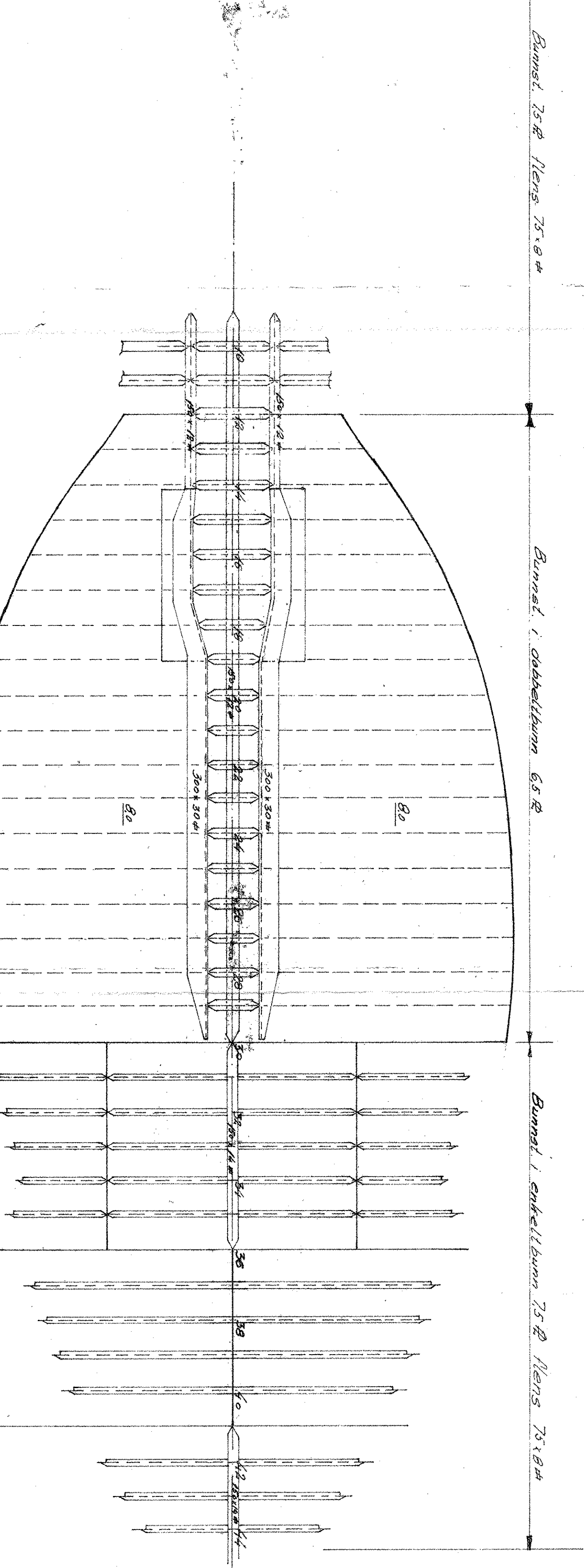
Bunnkonstruksjon "Moderfundament"
