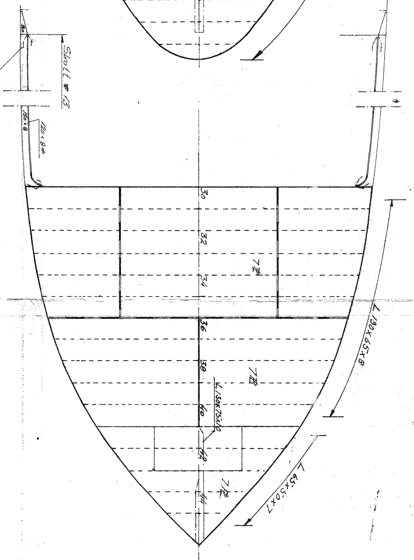
Innredningsdekk
