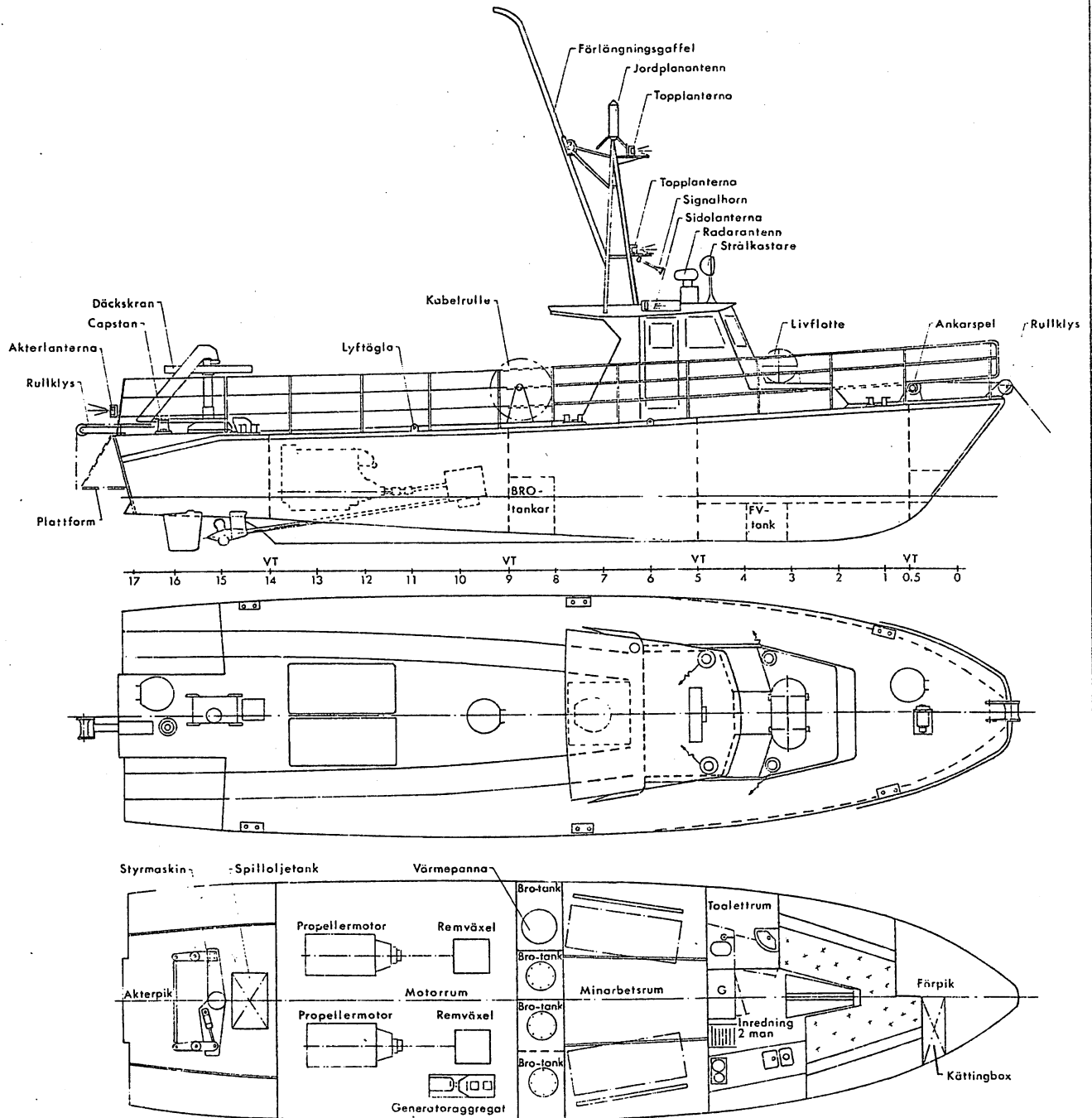
Bild 1 Arrangemang
